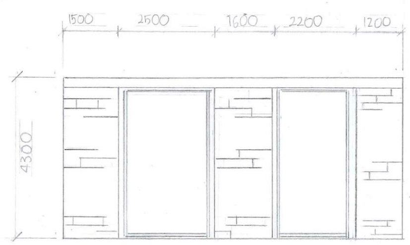
LH ELEVATION
